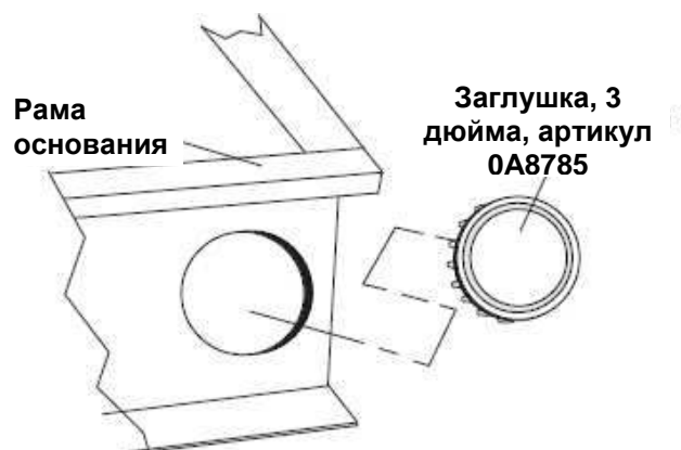
Рисунок 2.3. Заглушки рамы основания
