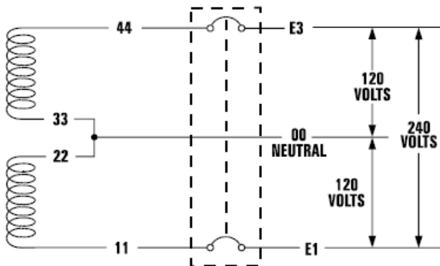
Рисунок 1.2. Статор 4 вывода, 1 фаза
